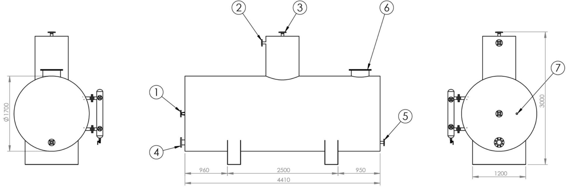
10 m 3 /h Deaazör Besi Tankı Montaj
